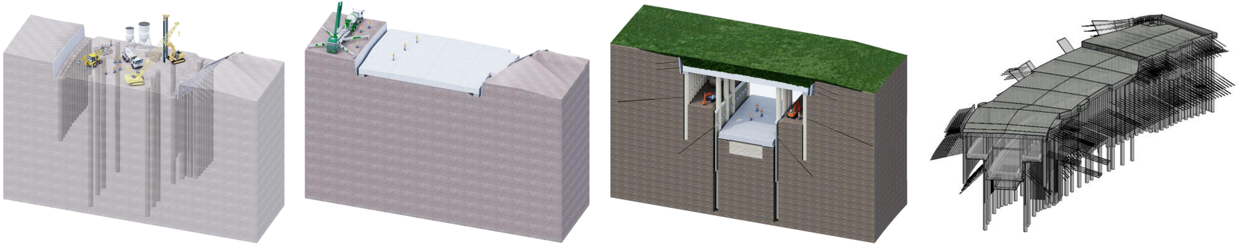
PRINCIPALI FASI ESECUTIVE (sopra) – DOCUMENTAZIONE FOTOGRAFICA (sotto) – MODELLO BIM (sopra a destra) – SEZIONE TRASVERSALE OPERA IN ESERCIZIO (sotto a destra)
